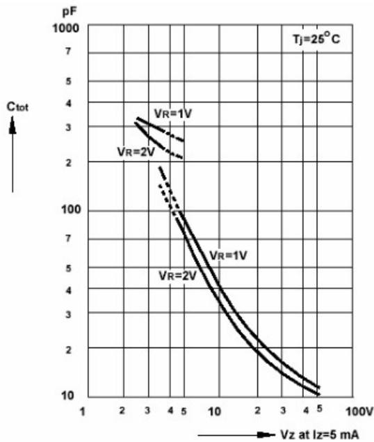
Capacitance versus Zener voltage
